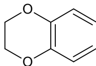
etylenodioksyfenyl-
